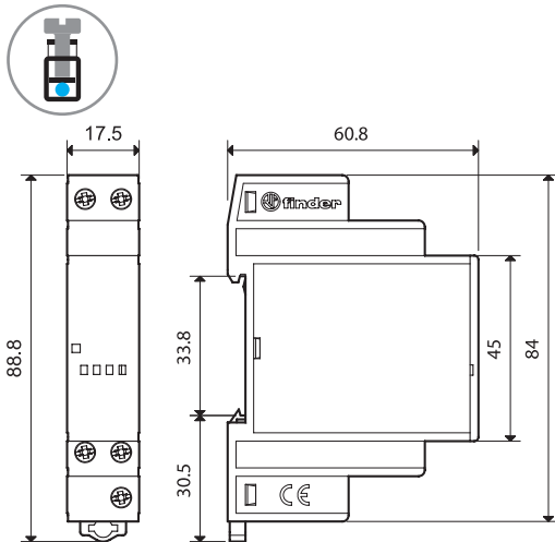
19.91 (módulo de potencia para 11.91) Borne de jaula
