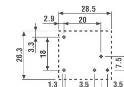
Vista parte inferior Largo de terminal 3.5 mm para CI o zócalos
