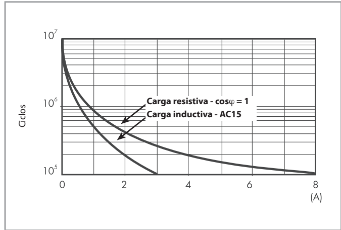
F 40.4 - Vida útil eléctrica (AC) en función de la carga Tipo 40.52 (página 3)
