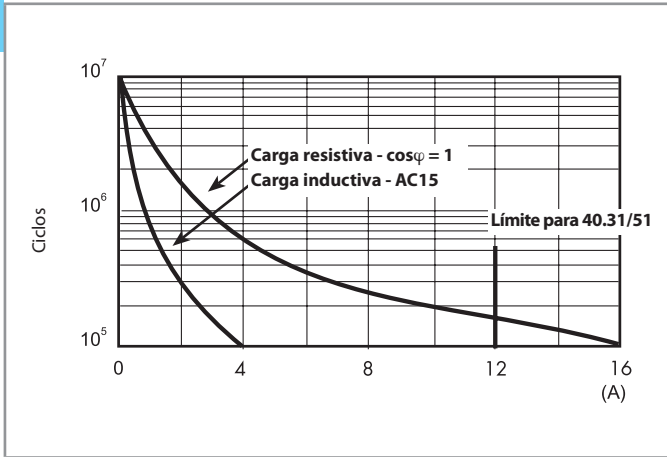
F 40.3 - Vida útil eléctrica (AC) en función de la carga Tipos 40.31/51/61 (página 3)
