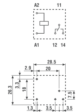
Vista parte inferior Largo de terminal 3.5 mm para CI o zócalos
