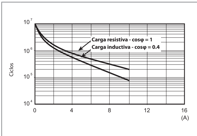
F 40.5 - Vida útil eléctrica (AC) en función de la carga Tipo 40.11
