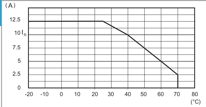
F L782E-1 Corriente de salida en función de la temperatura ambiente (78.2E)
