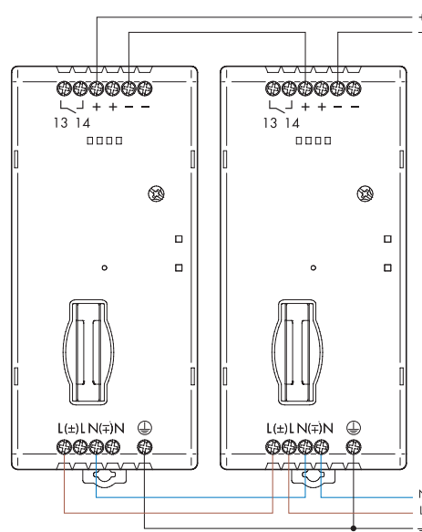
Conexión en serie
