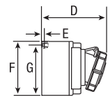
Entrelazado 20A, Vista Lateral
