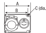
Entrelazado 20A, Vista Frontal
