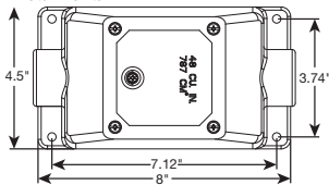
De Paso 20/23A y 30/32A Vista Frontal
