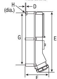
Entrelazado 20A y 30A Vista Lateral
