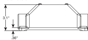
De Paso 20/23A y 30/32A Vista Lateral
