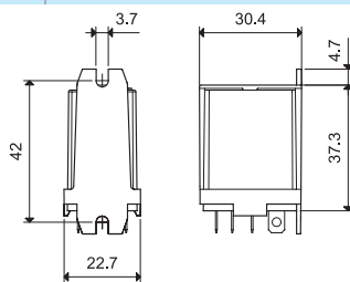
056.26 con relé
