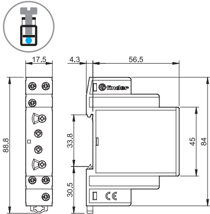
80.82 Borne de jaula
