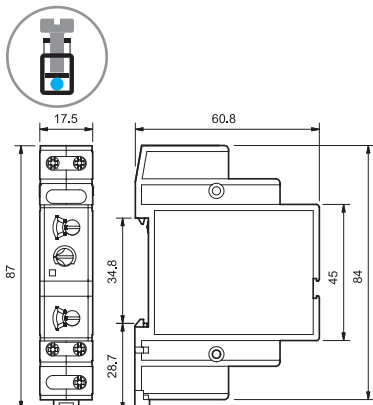
80.82 Borne de jaula
