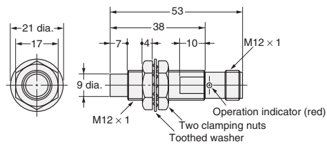
Fig. 22 : E2E-X5MY□-M1
