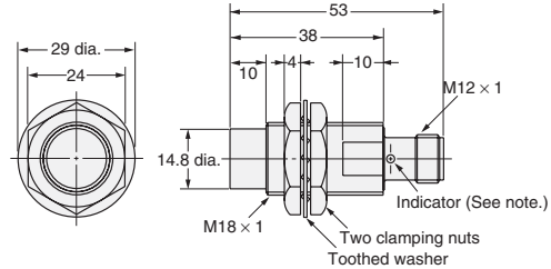
Fig. 24 : E2E-X14MD□-M1(G)/E2E-X10ME□-M1/F□-M1 E2E-X10MY□-M1
