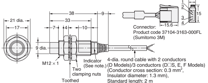
Fig. 9 : E2E-X8MD□ E2E-X5ME□/F□
