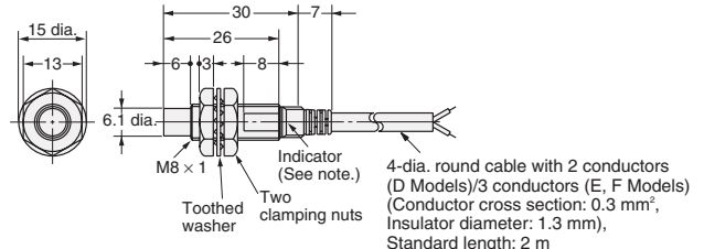
Fig. 5 : E2E-X4MD□ E2E-X2ME□/F□
